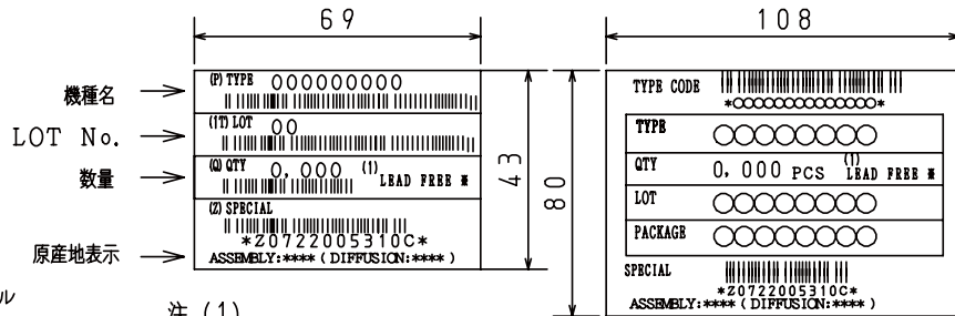
リールラベル, 内装箱ラベル (単位: mm)
