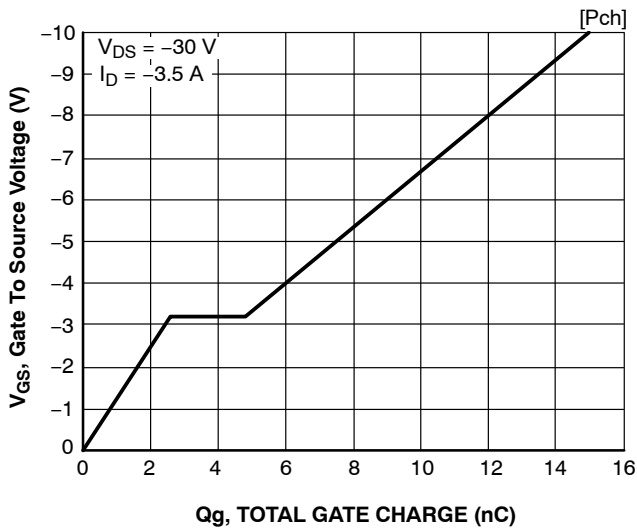
Figure 20. V_{GS} - Q_g
