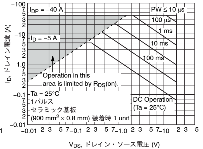
図 11. ASO
