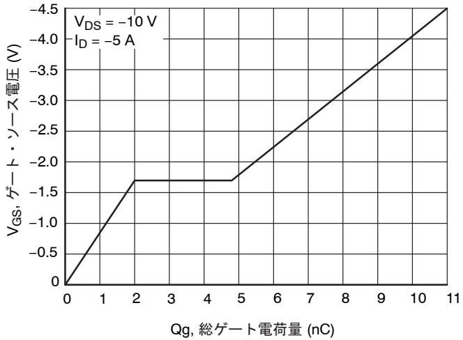
図 10. V_{GS} - Q_g
