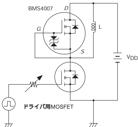
図3. 逆回復時間測定回路図
