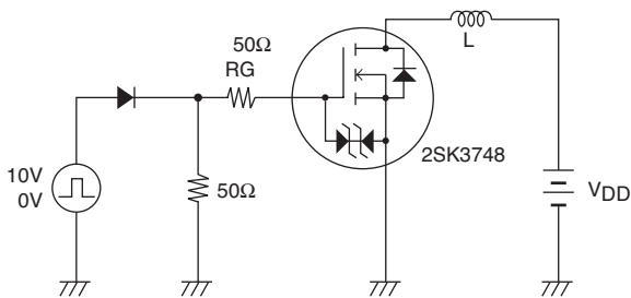
図 1. アバランシェ耐量測定回路図
