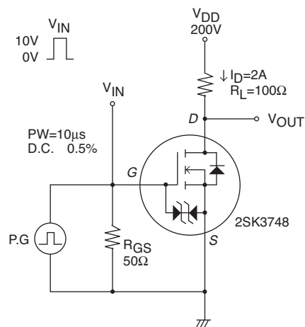
図 2. スイッチングタイム測定回路図
