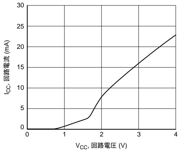
図 3. I CC - V CC
