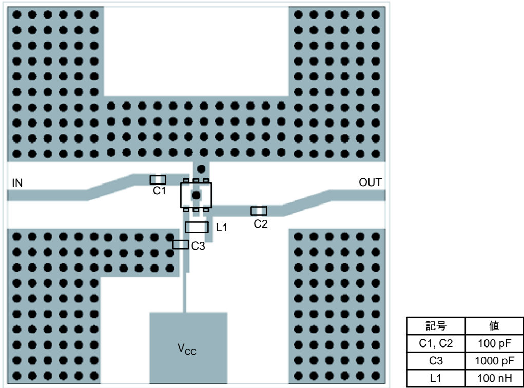
図 2. 評価基板
