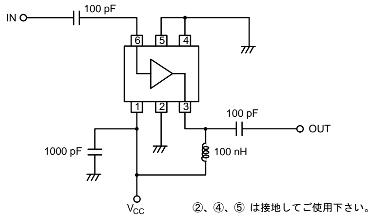
図 1. 測定回路図
