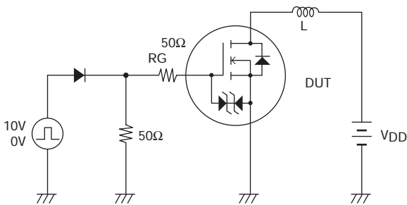
図 1. アバランシェ耐量測定回路図
