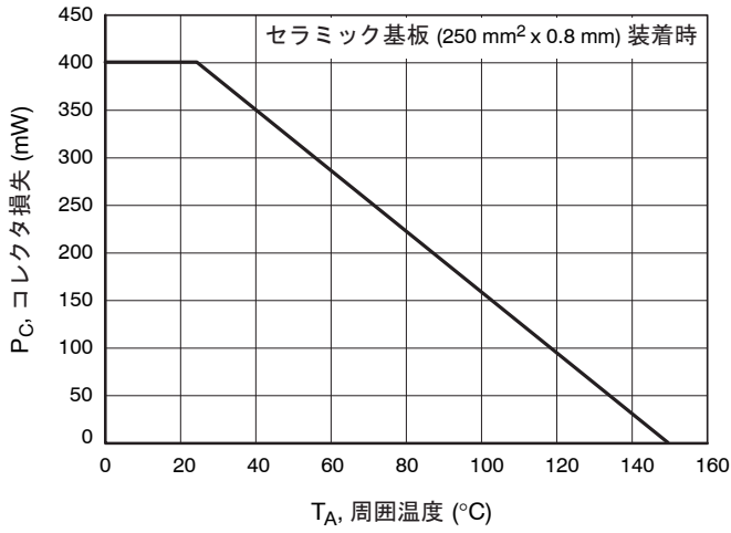
図 9. P_C - T_A
