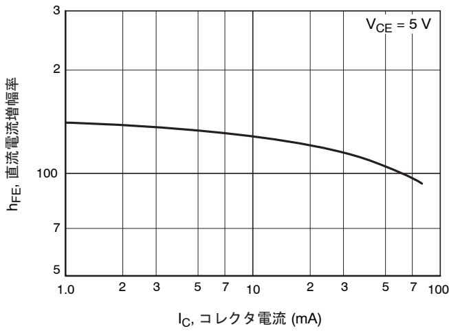
図 3. h_{FE} - I_C
