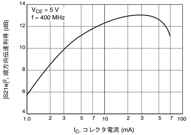
図 8. |S_{21e}|^2 - I_C
