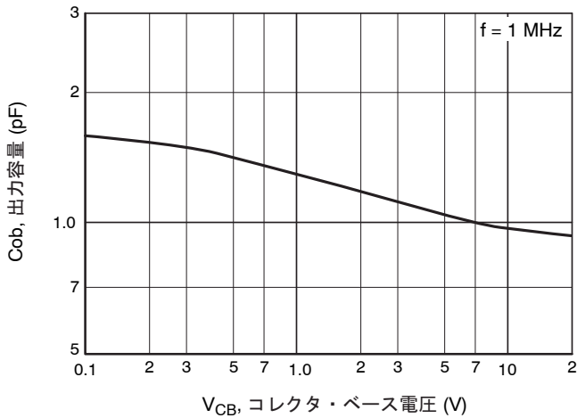
図 5. C_{ob} - V_{CB}
