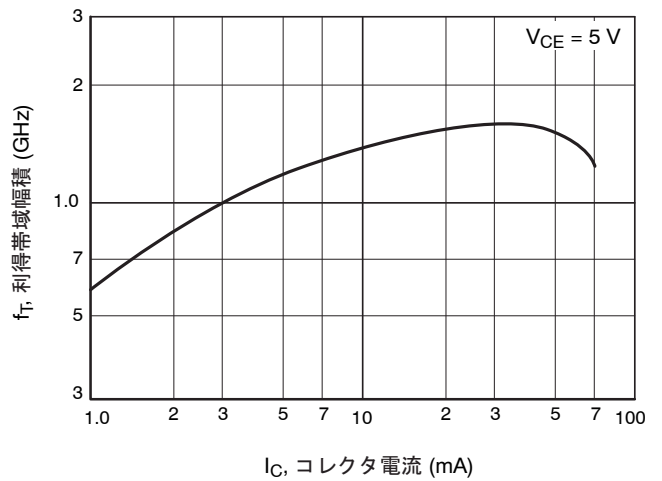
図 4. f_T - I_C
