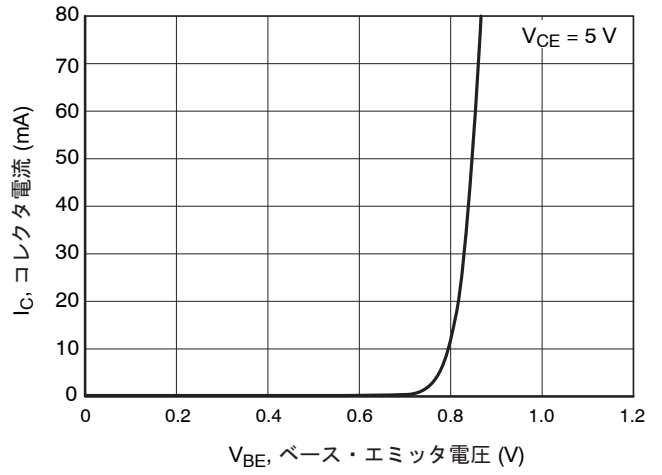
図 2. I_C - V_{BE}
