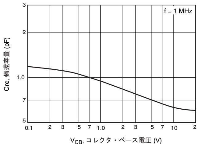
図 6. C_{re} - V_{CB}
