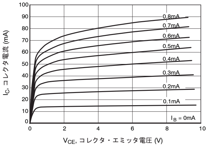
図 1. I_C - V_{CE}
