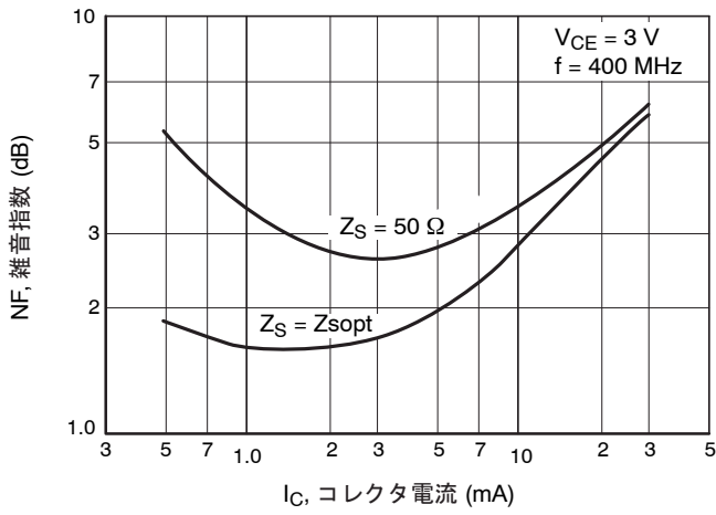
図 7. NF - I_C
